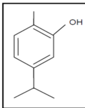
Figura 3. Estructura de carvacrol
