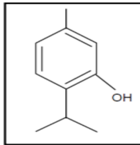
Figura 2. Estructura del Timol
